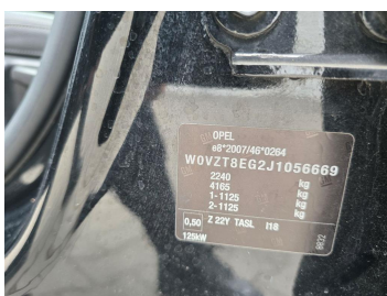
Tabliczka znamionowa
