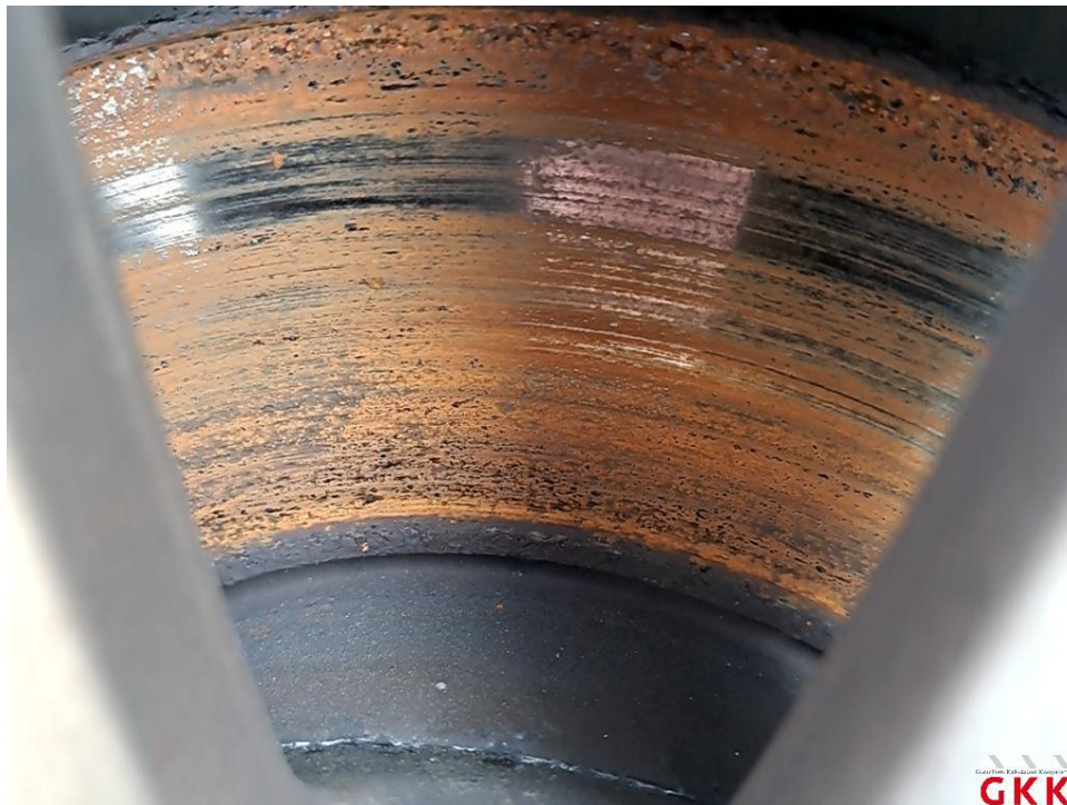
Bild 22 Bremsscheiben, vorne, korrodiert, ersetzen
