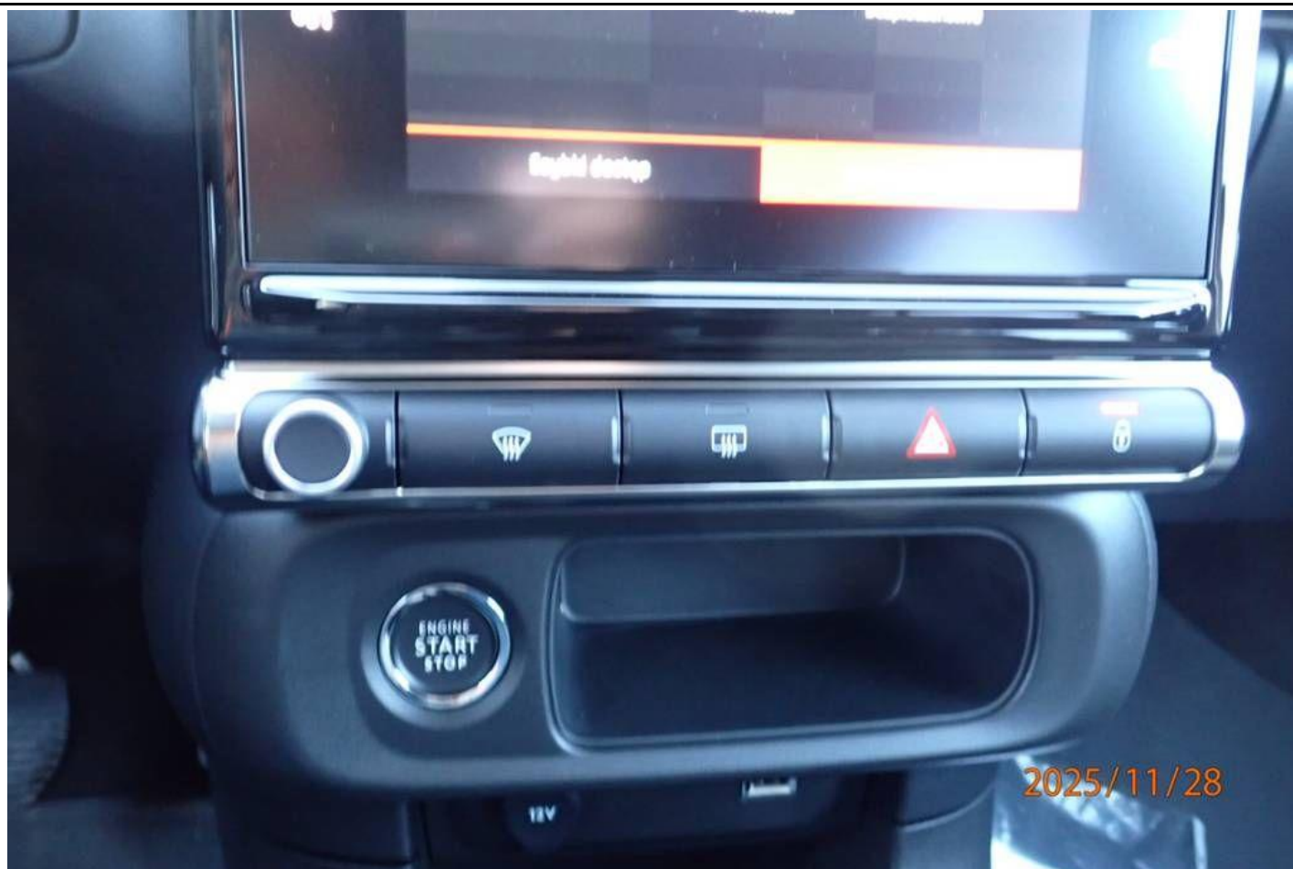
Fot. nr 103
