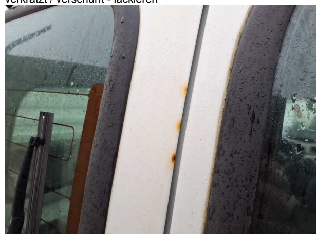
Beschädigung #19: Heckklappe/-tür: Hecktür links (Mit Rostbildung, inkl Leiste) - Lackmangel - instandsetzen und
