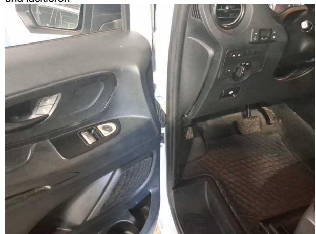
Beschädigung #8: Tür vorn links: Fangband / Feststeller - Geräusch - instandsetzen
