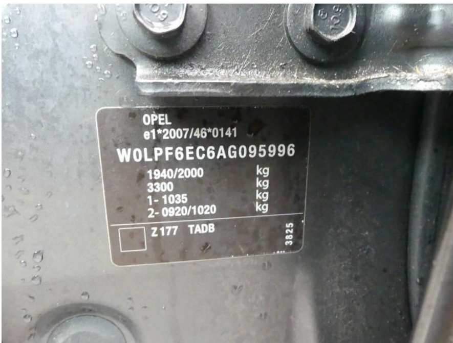
Bild 6: Fahrgestellnummer
