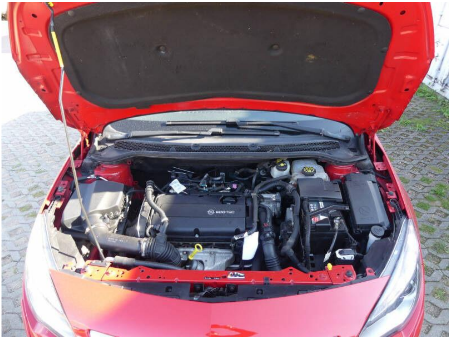
Bild 5: Motorraum
