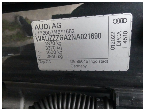
Bild 8: Typenschild
