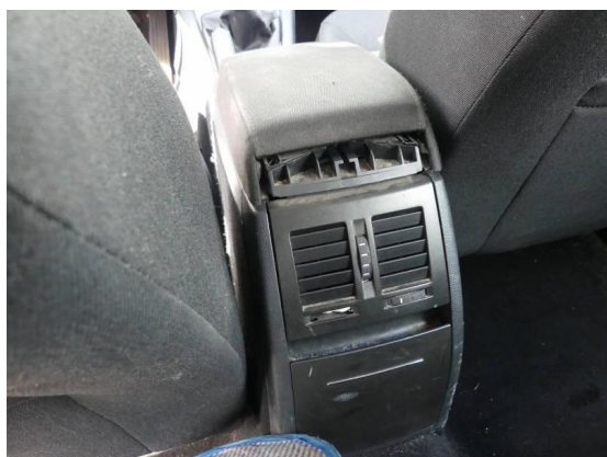
Bild 9: Innenraum / Drehregler Luftaustrittsdüse hinten links abgebrochen
