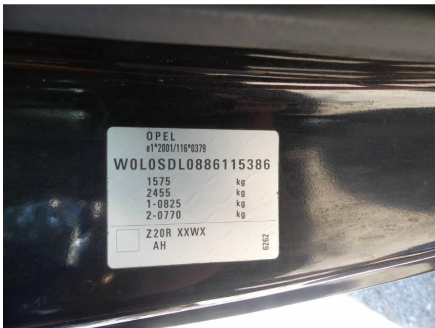
Bild 6: Fahrgestellnummer
