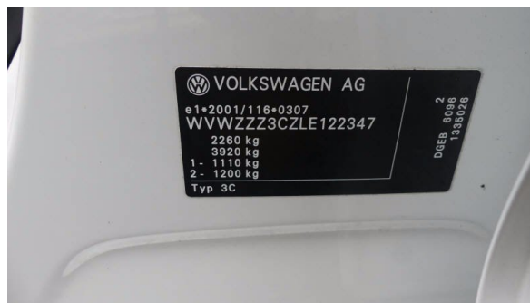
Bild 8: Typenschild
