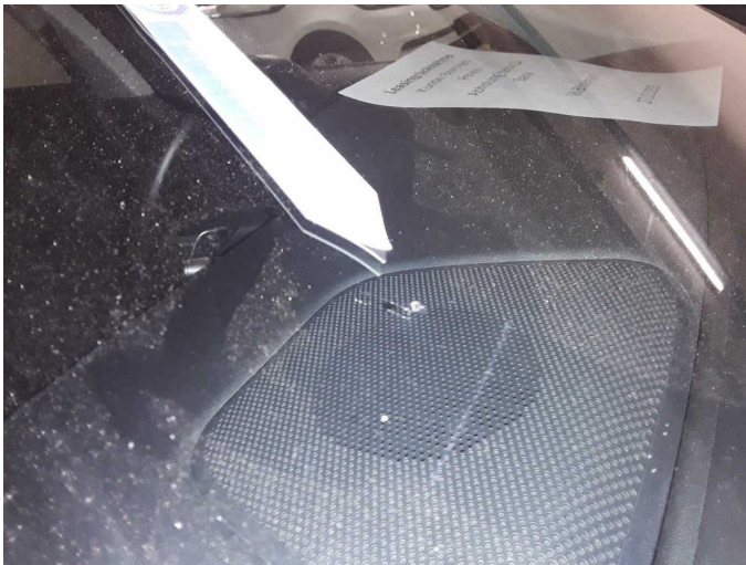
Beschädigung 2: Verglasung: Frontscheibe (mit Rissbildung) - Steinschlag - erneuern
