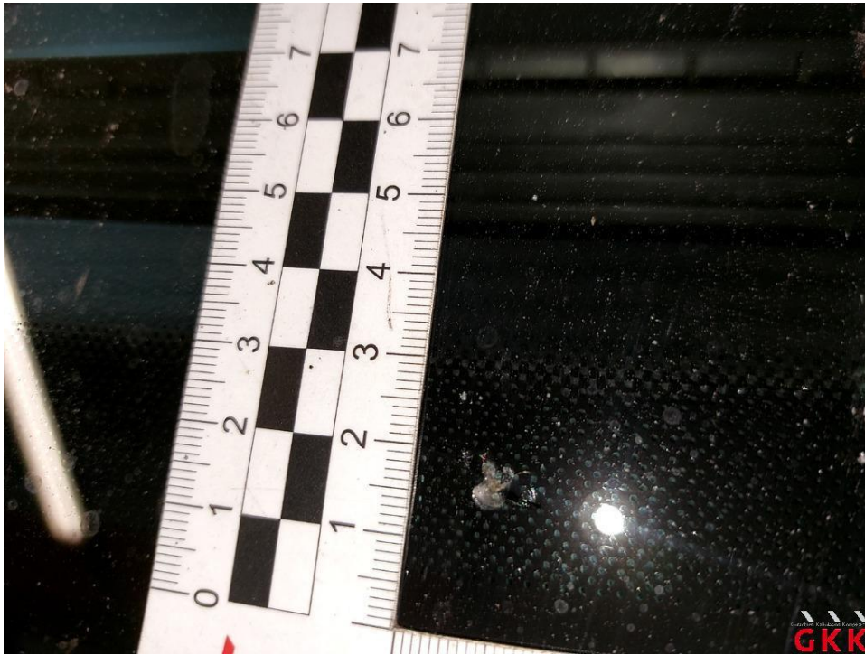
Bild 19 Frontscheibe, Steinschlag mit Rissbildung, ersetzen
