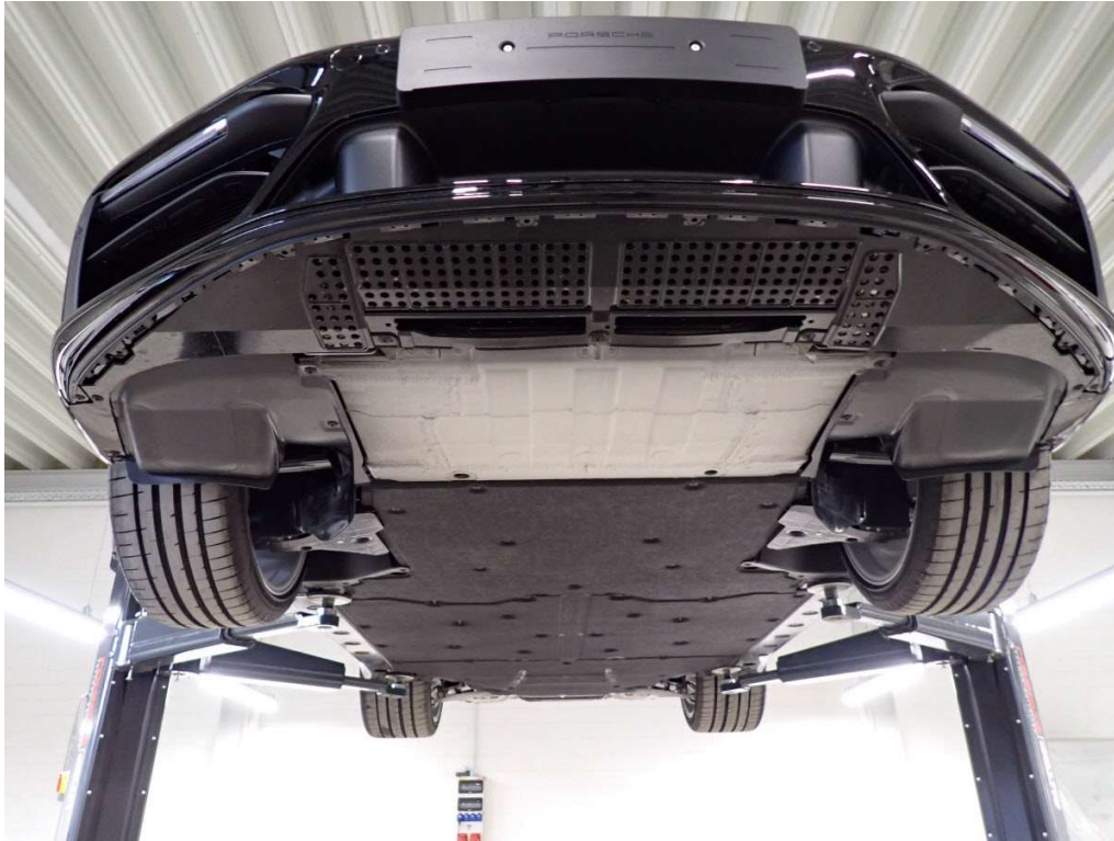
Bild 13 Unterboden vorn
